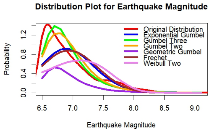
Fig. 11. Data 1:Earthquake magnitude
